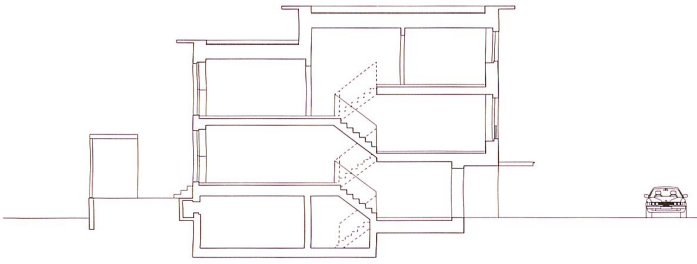
Reihenhaus, Schnitt
