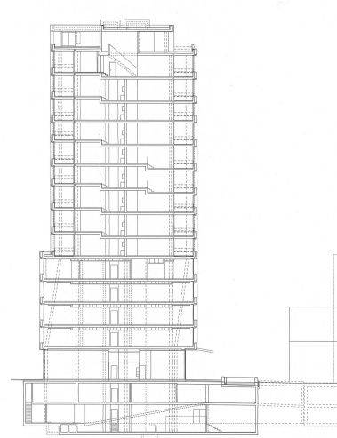
Schnitt
