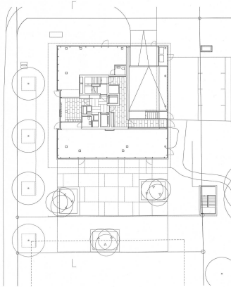
Erdgeschoss
