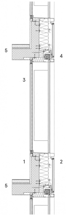
Konstruktionsschnitt vertikal
