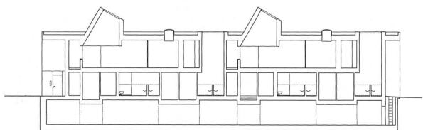
Schnitt A
