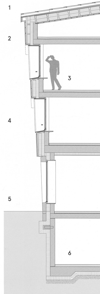
Detailschnitt
