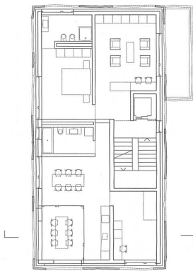
1. Obergeschoss
