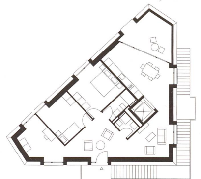
4. Obergeschoss
