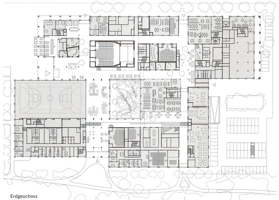
Erdgeschoss
