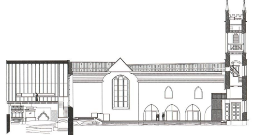
Längsschnitt
