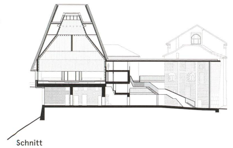
Schnitt
