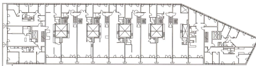
2. Obergeschoss
