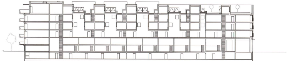
Schnitt
