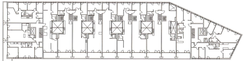
2. Obergeschoss
