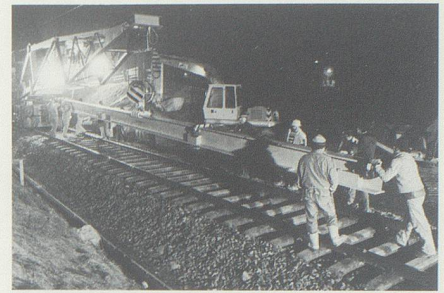
1./2. April: Die Bauarbeiten für die Bahnunterführung Bühel in Salez sind im Gange. Über Nacht wird eine Notbrücke erstellt.
