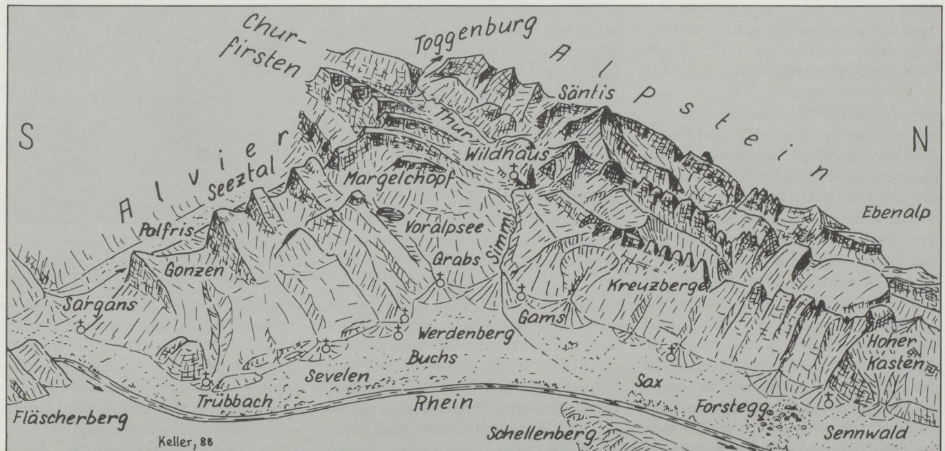
Figur 1: Blockbild von Alvier und Alpstein.
