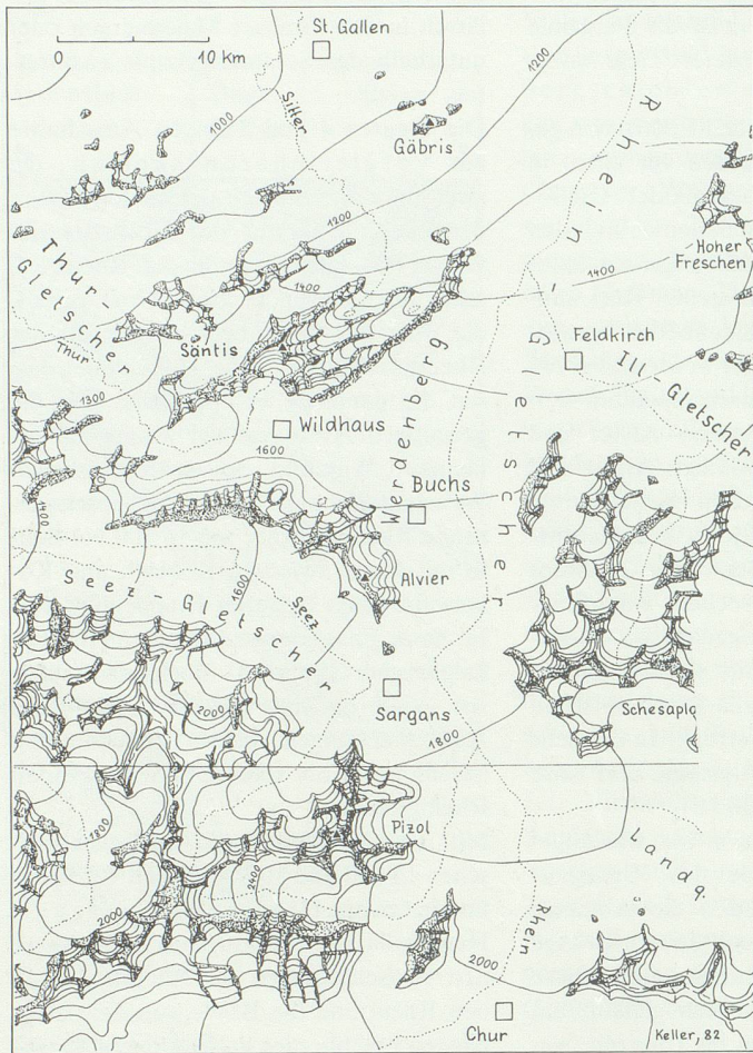
Figur 4: Der Rheingletscher im Maximum der letzten Eiszeit
