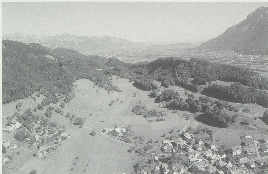
Bild 3: Die unteren Abhänge des Alvier sind, wie hier bei Oberschan, stark durch Gletschereis und Schmelzwasser überprägt worden. Während die Kuppen (meist bewaldet) eisgeschliffen sind, wurden die hangparallelen Tälchen in der Späteiszeit durch eisrandliche Wasserströme geschaffen (Bildmitte jeweils von rechts nach links).
