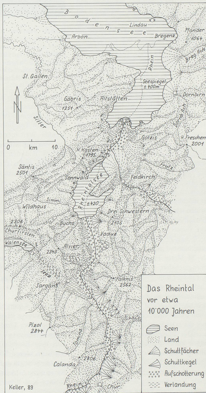
Figur 6: Die Alpengletscher waren um 10 000 J. v. h. bis ins Hochgebirge zurückgeschmolzen; ihre Ausmasse entsprachen den gegenwärtigen. Infolge Fehlens einer schützenden Pflanzendecke im Alpenraum war die Verfüllung des Rheintals rasch vorangeschritten. Der Ill-Schuttfächer hatte Bodensee und Rheintalsee voneinander getrennt. Gleichzeitig hatte der Rhein sein Delta von Bünden her bis Buchs vorgeschoben.
