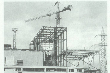
9. Juni: Die Ofenlinien 1 und 2 der Kehrichtverbrennungsanlage Buchs werden für rund 13,1 Millionen Franken nachgerüstet.
