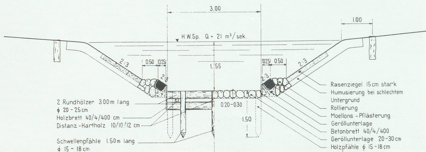
Beispiel eines symmetrischen, in erster Linie auf hydraulische Aspekte ausgerichteten Normalprofils aus dem Jahre 1958. Darstellung von Hansruedi Wildermuth in Maag 1989.
