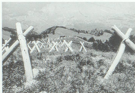
11. Juli: Zwischen dem Hohen Kasten und der Saxerlücke sind im Rahmen des Aufforstungsprojektes Sennwald bisher 1756 Dreibeinböcke angebracht worden.
