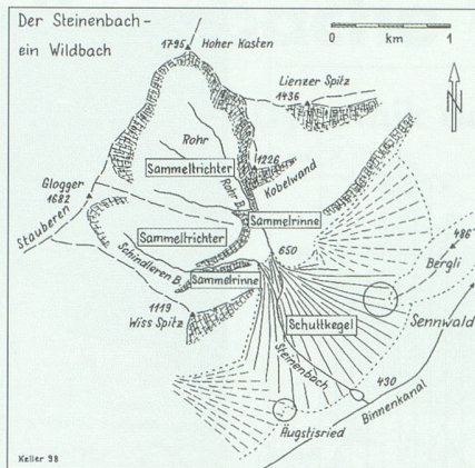
Figur 4: Der Steinenbach mit seinen zwei Quelllästen weist in muster-gültiger Art und Weise die Hauptmerkmale von Wildbächen, nämlich die drei Abschnitte Sammeltrichter, Sammelrinne und Schuttkegel auf.
