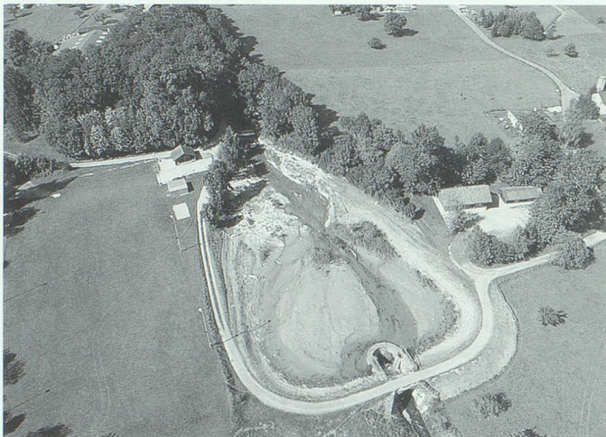
Der Kiessammler des Steinenbachs in Sennwald. Er wurde um 1906 beim Bau des Rheintaler Binnenkanals erstellt. Bild 1994: Hans Jakob Reich, Salez.
