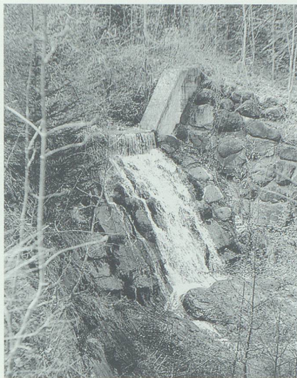
Kolkschutz (Energievernichter) nach einer Betonsperre im Walchenbach, Grabs. Bild: Eugen Henauer, Buchs.
