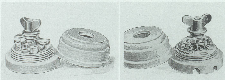
Schalter für Innenanlagen, um 1900, links mit Zungenkontakten, rechts mit Bürstenkontakten. Die Platten und Deckel waren aus Porzellan. Die Schalter konnten in beliebiger Richtung gedreht werden. Wyssling 1946
