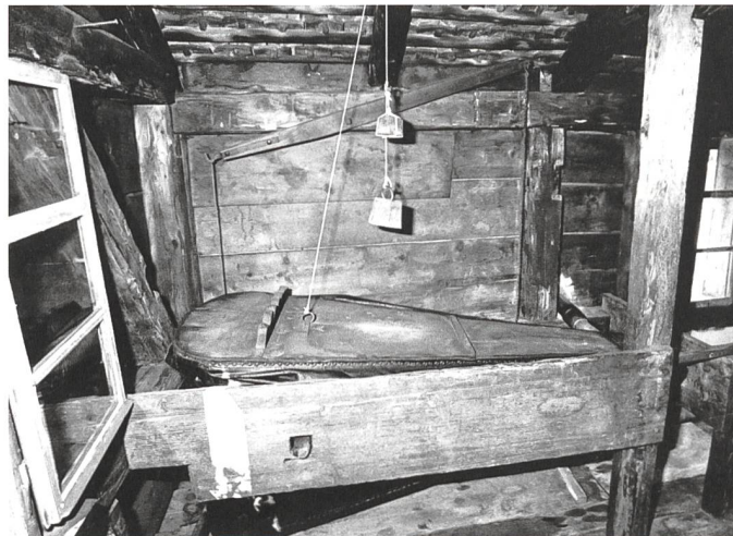
2. Mai 1987: Der alte Blasebalg in seiner ursprünglichen Form am alten Standort am Farbbach.
