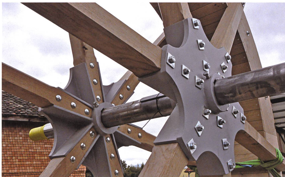
11. Juli 2012: Wichtiges Detail am neuen Wasserrad der Messerschmitte.
