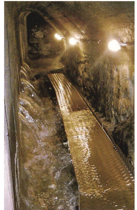
In der Quelffassung Fermärsch tritt das Wasser in zwei horizontalen Spalten aus dem Fels. Foto EW Azmoos
