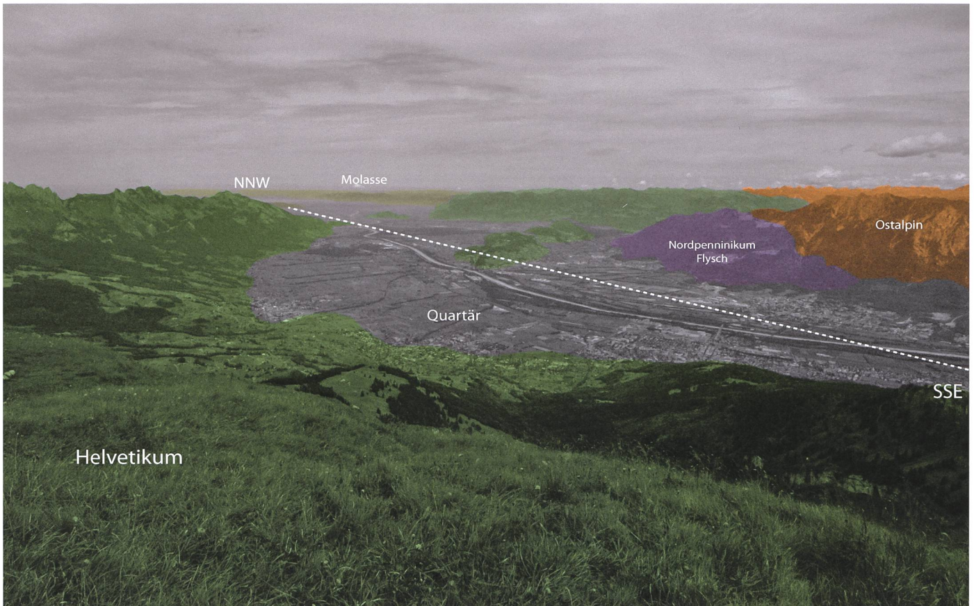
Abb. 14. Blick Richtung Norden von Imbabun ins Rheintal. Die helvetischen Decken (grün), vorwiegend aus der Kreidezeit, sind von Südosten her von den Flyschden der penninischen Decken überschoben, die aus oberer Kreide und Tertiär stammen. Diese wiederum sind ebenfalls von Südosten her von den weitaus älteren ostalpinen Decken der Trias überschoben.
