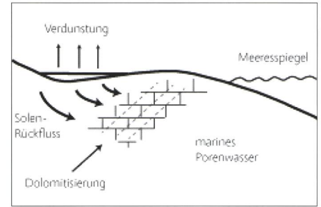
Abb. 7. Dolomitisierung: In bereits vorhandene Kalkablagerungen drangen salzreiche Solenflüsse aus Verdunstungströgen ein. Dabei wurde dem Kalk Magnesium eingelagert: Der Kalk wurde zu Dolomit umgewandelt.
