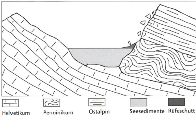
Abb. 6. Vereinfachter Querschnitt durch das Rheintal (West–Ost).
