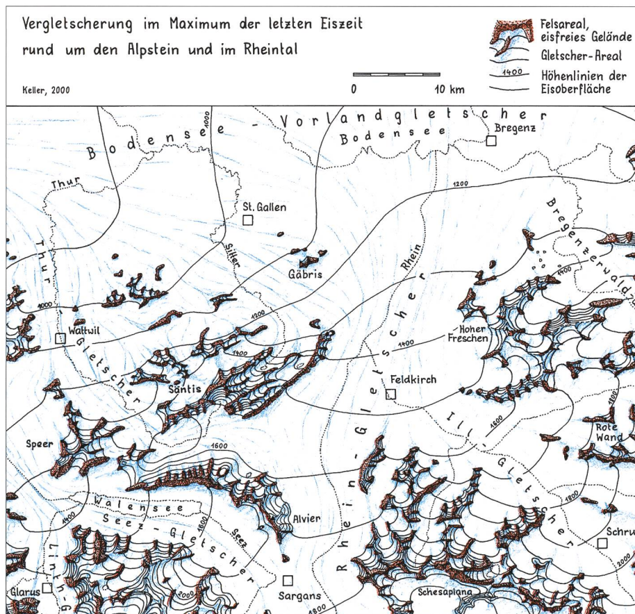
Abb. 18. Der Alpennordrand und das Bodenseegebiet vor 20 000 Jahren. Aus Keller 2009 Der mächtige Rheingletscher verzweigte bei Sargans in den Seezgletscher ab. Bei Feldkirch floss er mit den Gletschern der Vorarlberger Alpen zusammen und breitete sich im Bodenseebecken aus. Nur die höchsten Gebirgsketten wie Dreischwestern, Alpstein und Churfirnen ragten wie Inseln aus dem zusammenhängenden Eisstromnetz heraus. Die Höhenkurven zeigen die Höhenlagen der Eisoberfläche. Im Liechtensteiner Rheintal lag sie zwischen 1400 und 1800 m ü. M.
