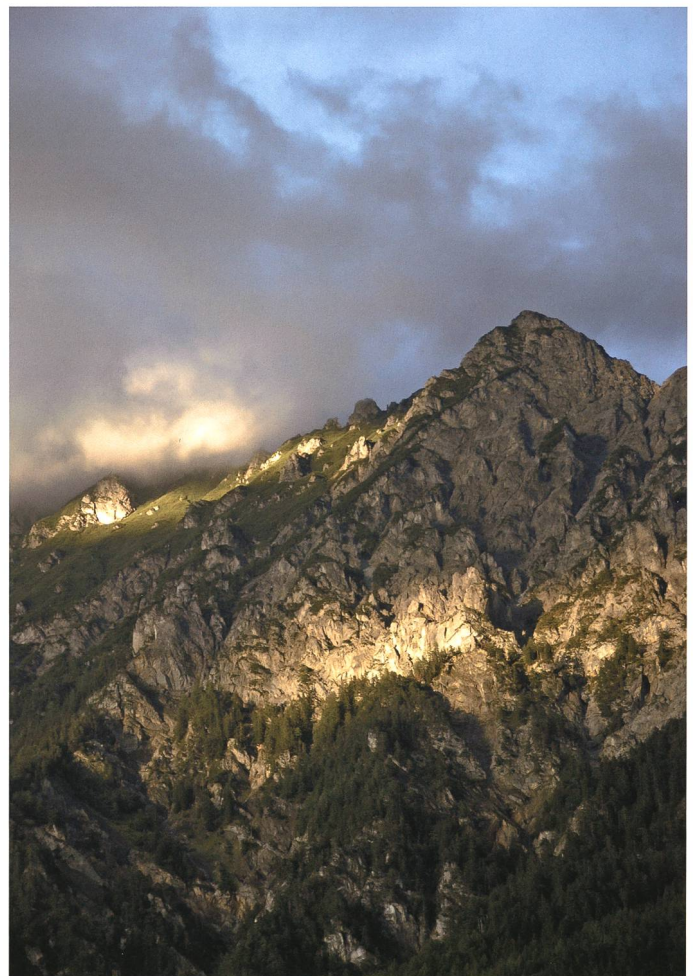
Abb. 8. Der schroff verwitterte Hauptdolomit der Dreischwesternkette ist das dominante gipfelbildende Gestein der Liechtensteiner Rheintalseite. Zur Triaszeit, vor rund 250 Millionen Jahren, wurde er im sehr seichten Wasser der südlichen Randmeerbereiche der Tethys gebildet.
