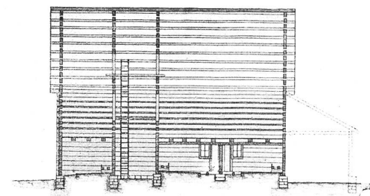
Längsschnitt
