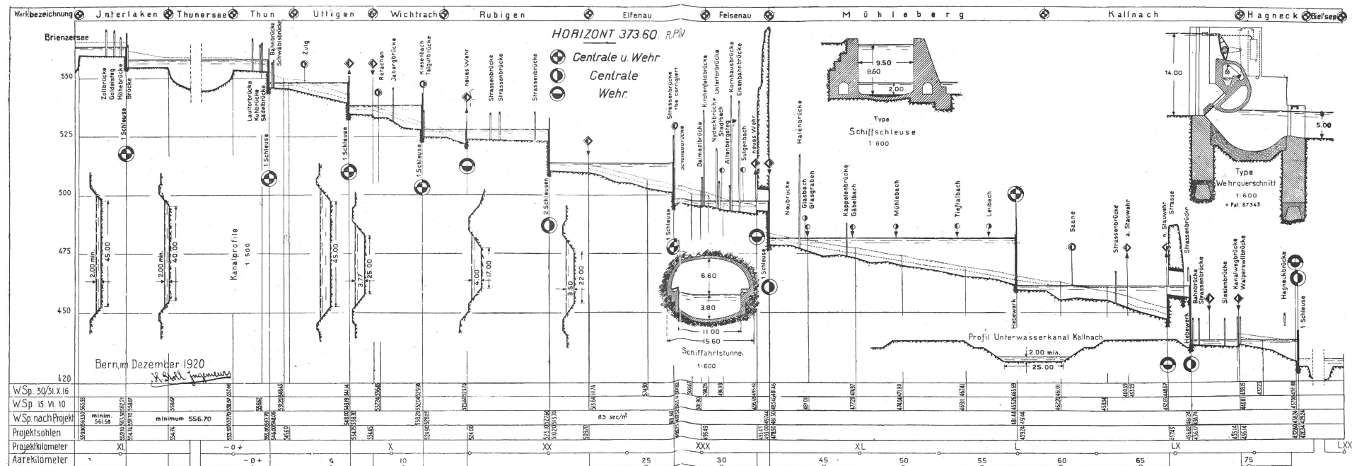
Wasserwirtschaftsplan des ober Aaregebietes bis zum Bielersee.
