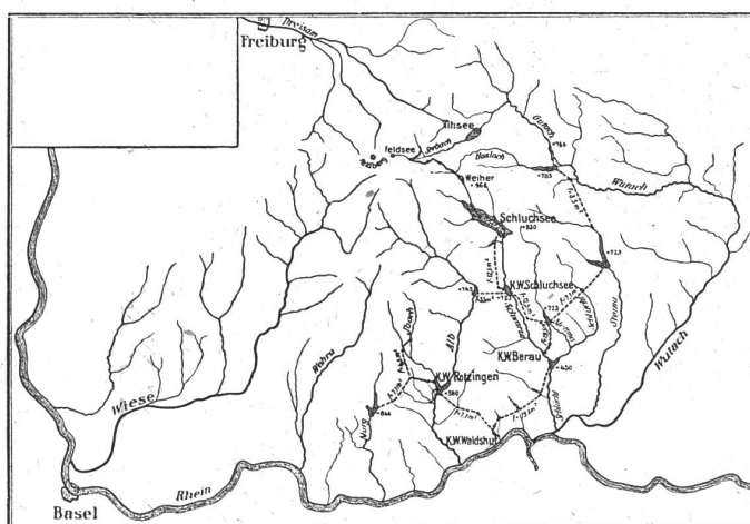
Abb. 5. Übersichtslegeplan - Entwurf „Kettenwerke“.
