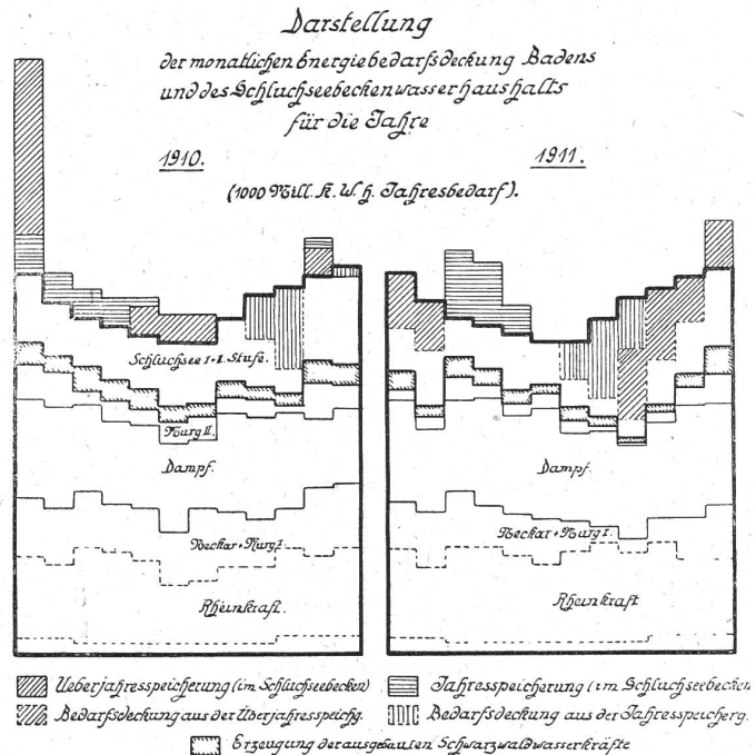
Abb. 17. Darstellung der monatlichen Energiebedarfsdeckung Badens und des Schluchseebeckenhaushalts.
