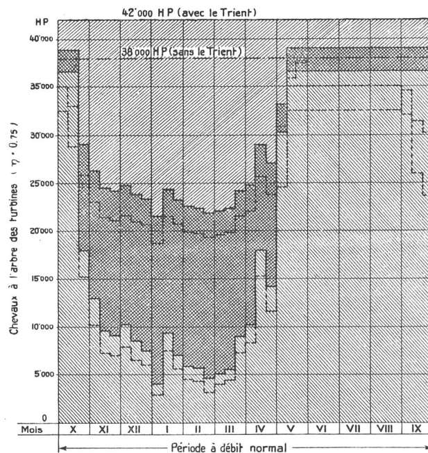
Abb. 1. Zusammenarbeit der Kraftwerke Barberine und Vernayaz.
