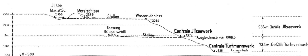
Abb. 6. Illsee-Turtmann. Längenprofil. Höhen- und Längen-Maßstab 1 : 100 000.
