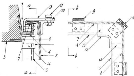
Abb. 1. Schnitt b-b
