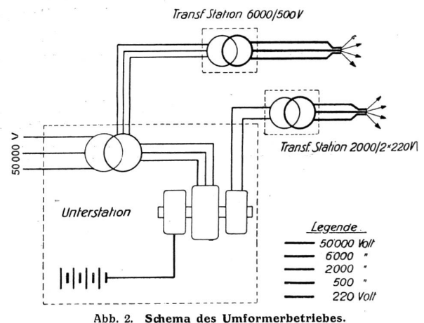
Abb. 2. Schema des Umformerbetriebes.
