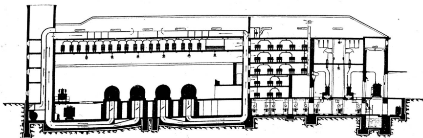
Abb. 6. Schnitt durch die Zentrale Neu-Selnau (im Bau).
