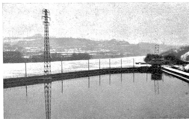
Abb. 38. Kraftwerk Laufenburg. Blick vom Werk ins Oberwasser Februar 1929.
