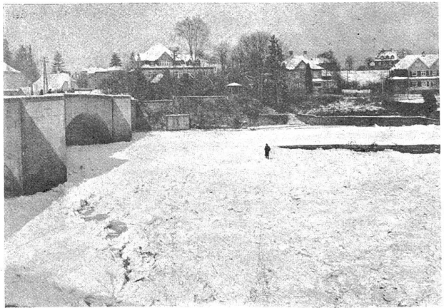
Abb. 50. Kraftwerke Augst-Wyhlen. Packeisbildung oberhalb der Rheinbrücke in Rheinfelden. Februar 1929.
