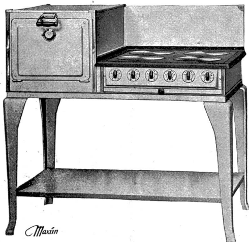
Abb. 2. Der neue Haushalterd der Maxim A. G., Aarau Backofen seitlich.
