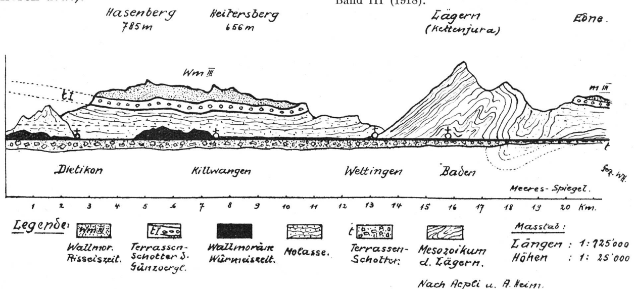
Abb. 4. Längsprofil durch das untere Limmattal.
