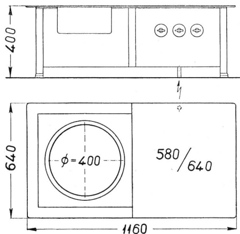
Abb. 50 Hochleistungs-Kochstelle Fabrikat: Zahler & Co., Biel
