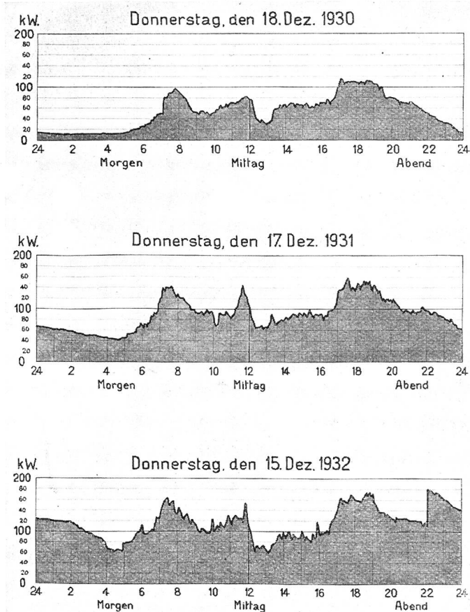
Abb. 12 EW Uzach. Belastungskurven in drei aufeinanderfolgenden Jahren.
