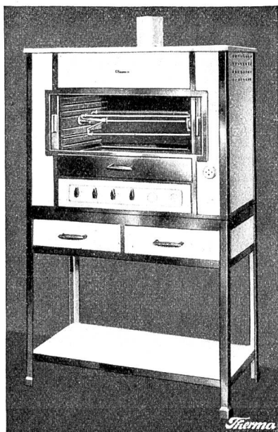
Fig. 10 Grill mit Jalousieverschluss und eingebautem Drehspieß
