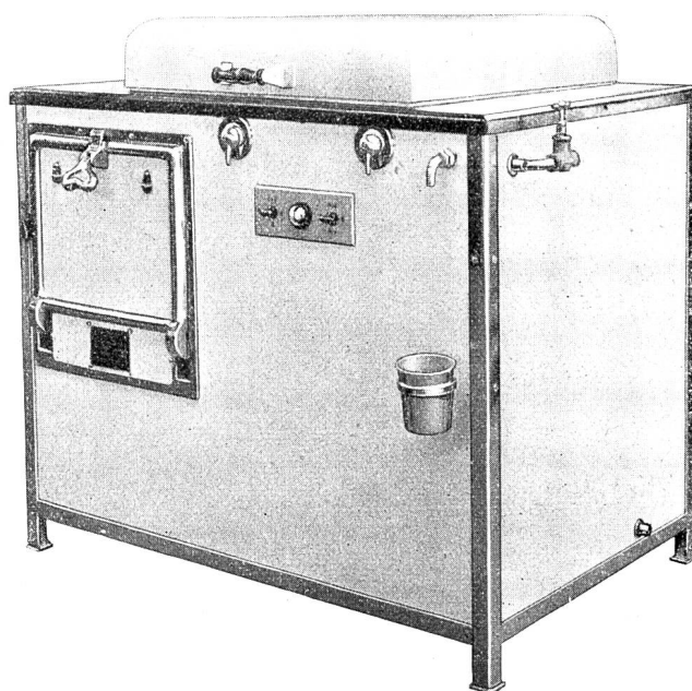
Fig. 9 Pilum-Speicherherd mit 2 Platten, Backofen und Boiler Cuisinière à accumulation «Pilum», à deux plaques, four et réservoir d'eau chaude (A.G. der Eisen- und Stahlwerke vorm. Georg Fischer, Schaffhausen.)
