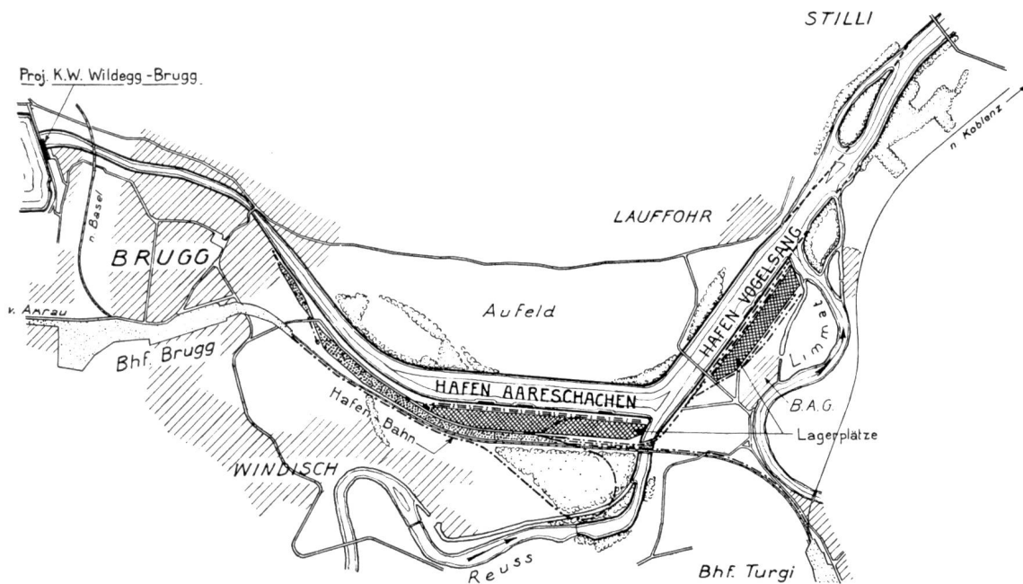
Abb. 16 Hafenanlage Brugg (Projekt A.) Hafenbecken bei Vogelsang und im Aareschachen. Regulierung der Aare vom Stauende Beznau bis zur Mündung der Reuss. Verlegung der SBB.-Linie zwischen Brugg und der Reussbrücke. Situationsplan Maßstab ca. 1:36.000
