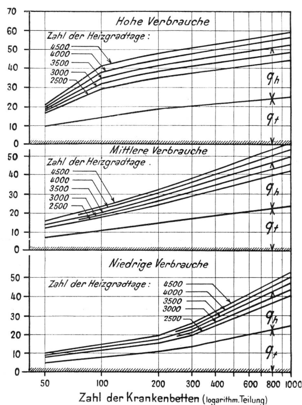
Abb. 61 Spezifische Wärmeverbräuche
