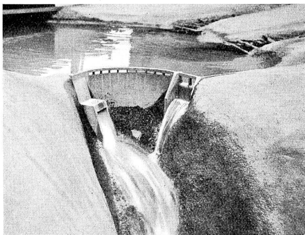
Abb. 4 Das Wasserbaumodell. Staumauer der Hochdruckanlage. Versuchsanstalt für Wasserbau an der E.T.H.
