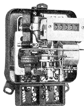
Fig. 7 Einphasen-Spitzenzähler mit einstellbarem mechanischem Gegendrehmoment (Landis & Gyr, Zug).
