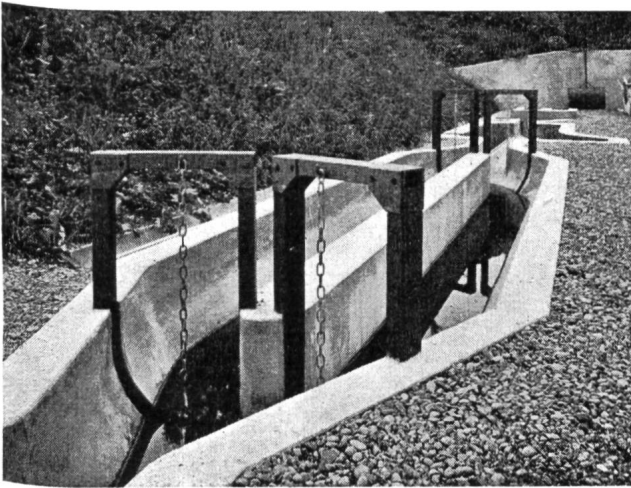
Abb. 4 Ansicht des Sandfanges, gegen Fliessrichtung gesehen.
