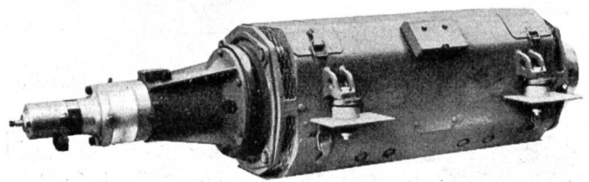
Abb. 4 Triebmotor, Aussenansicht.
