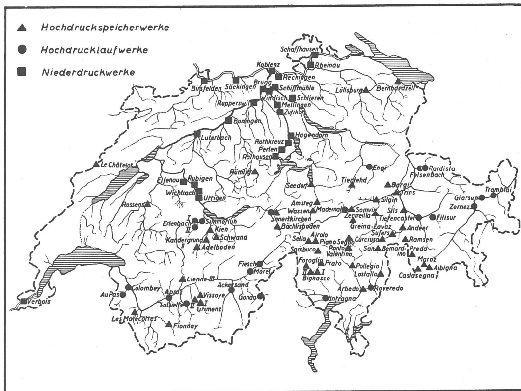
Abb. 1 Projektierte ausbauwürdige und im Bau befindliche Wasserkraftwerke in der Schweiz mit einer Ausbauleistung von mindestens 5000 kW (Stand Anfang 1941). (Nur Speicherwerke mit Gestehungskosten der Winterenergie von höchstens 6 Rp./kWh berücksichtigt).
