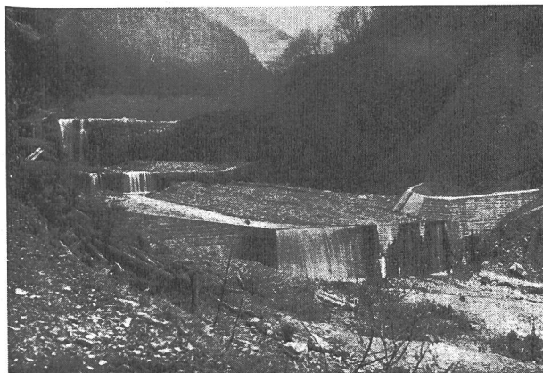
Abb. 7 Nollaverbauung. Sperre II mit Vorsperre und neuer Sperre. (Nr. 5045 BRB 3. X. 1939)
