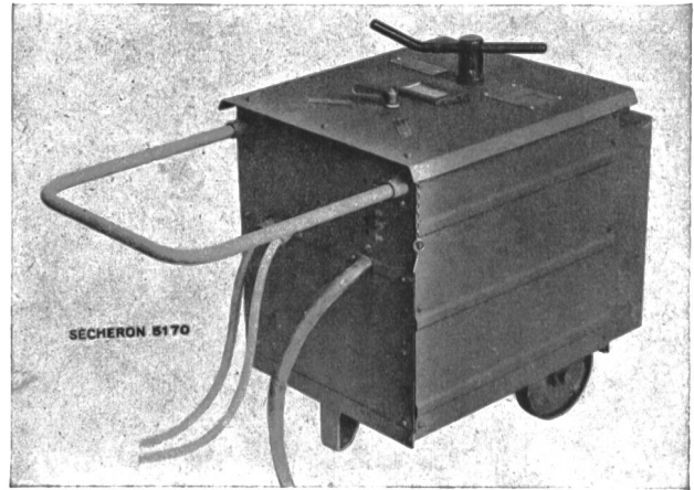
Fig. 31 Sécheron-Schweißapparat Typ SC 170 mit stufenloser Regulierung des Schweißstromes. Appareil à souder Sécheron type SC 170 avec réglage continu du courant de soudure.
