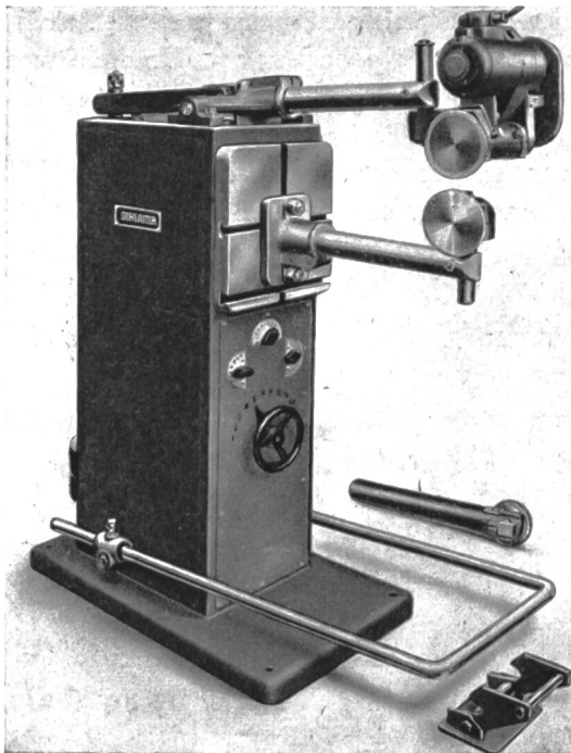
Fig. 30 Nahtschweißmaschine (A.-G. vorm. H. A. Schlatter & Co., Zollikon). Machine à souder par traits (S.A. ci-devant H. A. Schlatter & Co., Zollikon).
