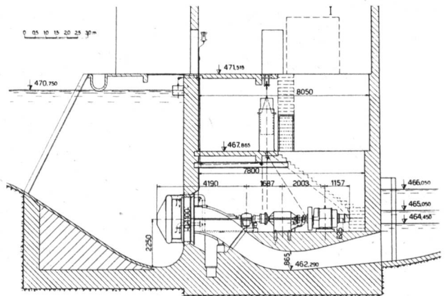
Abb. 17 Ersatz der in Abb. 16 gezeigten Turbine durch eine horizontalaxige Kaplan turbine mit Antrieb des Generators durch Spezialstirnräder. Diese Turbine ist gebaut für: Gefälle 4,7–5,7 m, Wassermenge 3460–5700 l/sek, Leistung 193–360 PS, Drehzahl 233–383 UpM. Auf Anregung des Wasserkraftbesitzers wurden die Turbinendimensionen für beste Ausnützung kleiner und kleinster Wassermengen gewählt. Dank des Spezialgetriebes der S. L. W. kann durch stufenweise Steigerung der Turbinendrehzahl der Wasserdurchlass der Turbine nach Bedarf bis zu 44% und damit deren Leistung um 65% gesteigert werden. Man beachte ferner die hydraulisch günstige Form des Turbinenauslaufes.
