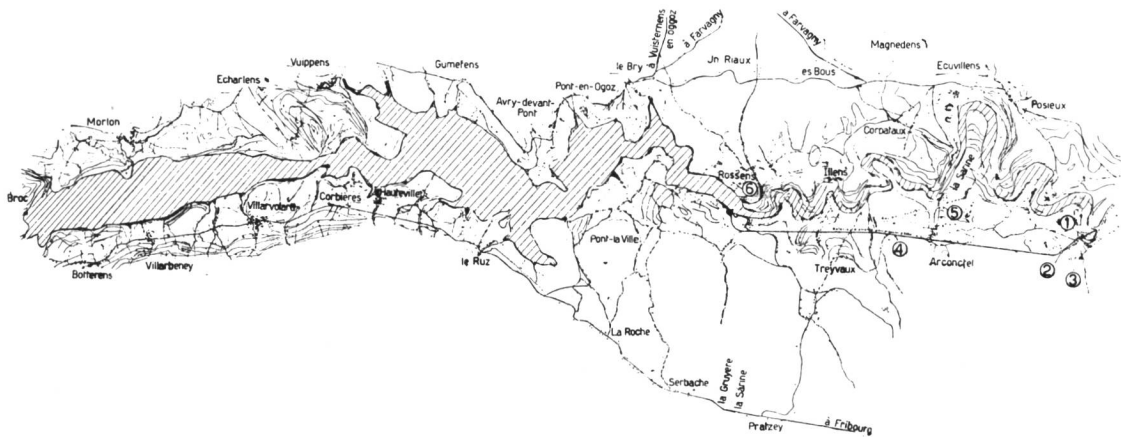
① Kraftwerk Hauterive, ② Wasserschloss, ③ Fenster, ④ Druckstollen, ø 5,0 m, ⑤ bestehender Stollen, ⑥ Staumauer.
