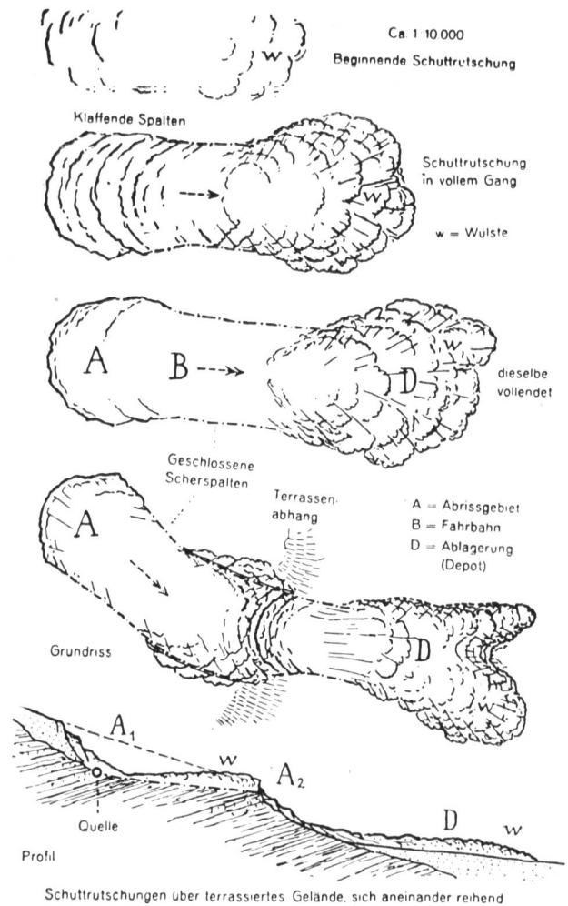
Schuttrutschungen über terrassiertes Gelände, sich aneinander reihend Abb. 19 Verschiedene Phasen von Schuttrutschungen. (Nach: Alb. Heim, Bergsturz und Menschenleben, 1932)
