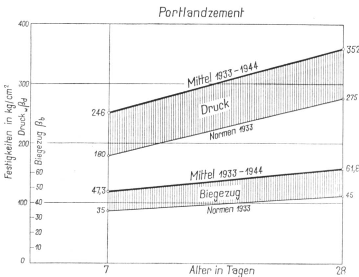
Abb. 4 Schweizerische Portlandzemente (PZ) 1933 bis 1944. Gesamtmittelwerte der Biegezug- und Würfeldruck-Festigkeiten. Alter 7 und 28 Tage. Normenwerte 1933.
