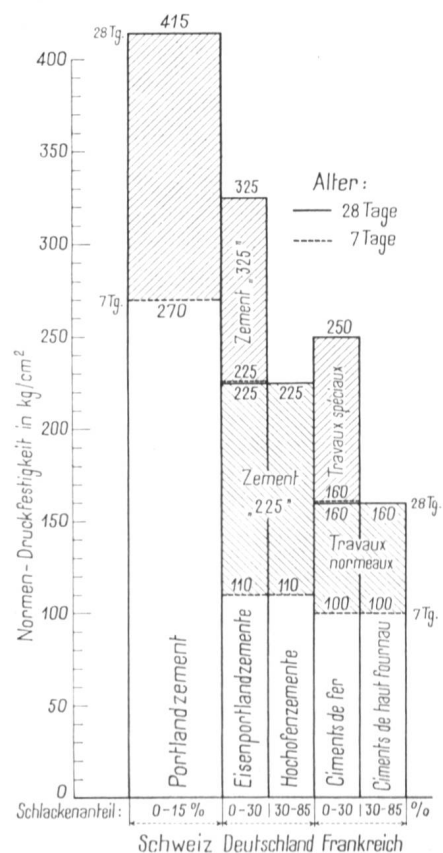
Abb. 1 Normen-Druckfestigkeiten. Portlandzement mit Zuschlägen von Schlacke. Schweiz, Deutschland, Frankreich. Mörtel 1:3, Gemischtkörniger Sand, Konsistenz plastisch. — Schweiz, Schlackenzement: Normendruckfestigkeit im Alter von 28 Tagen \approx rd. 220 kg/cm 2 . SIA-Normen 1933: Normensand: \approx rd. 150 kg/cm 2 .
