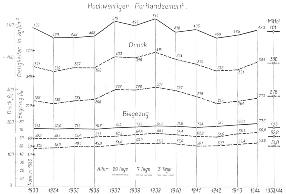
Abb. 5 Schweizerische hochwertige Portlandzemente (HPZ) 1933 bis 1944. Biegezug- und Würfeldruck-Festigkeiten. Jahresmittelwerte. Gesamtmittelwerte. Alter 3, 7 und 28 Tage. Normenwerte 1933.
