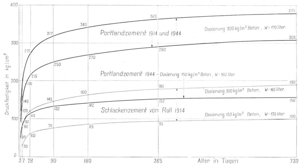
Abb. 2 Beton. Schweiz. Portlandzemente 1914 und 1944 und Schlackenzement von Roll 1914. Würfeldruckfestigkeiten w\beta_d . Dosierungen: 150 und 300 kg/m 3 . Konsistenz plastisch. Alter bis 2 Jahre.
