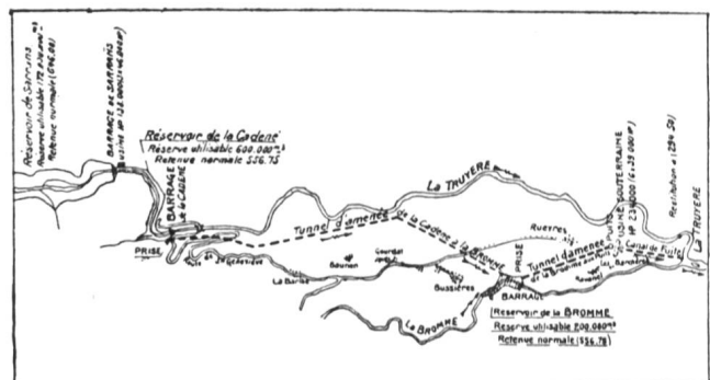
Lageplan der Truyère-Kraftwerke
